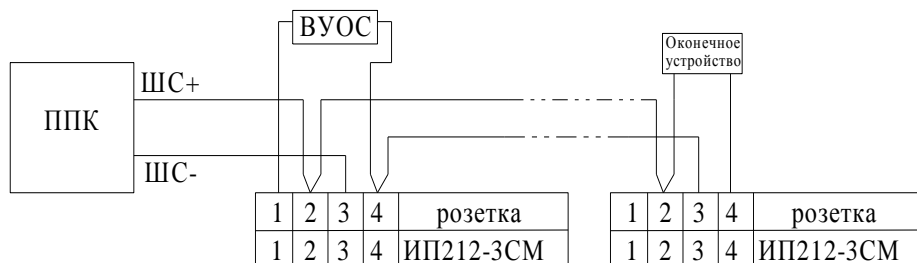
Рисунок 1 – Схема включения.
