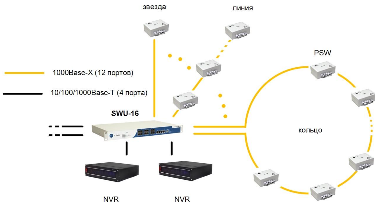
Рис. 1. Схема подключения
